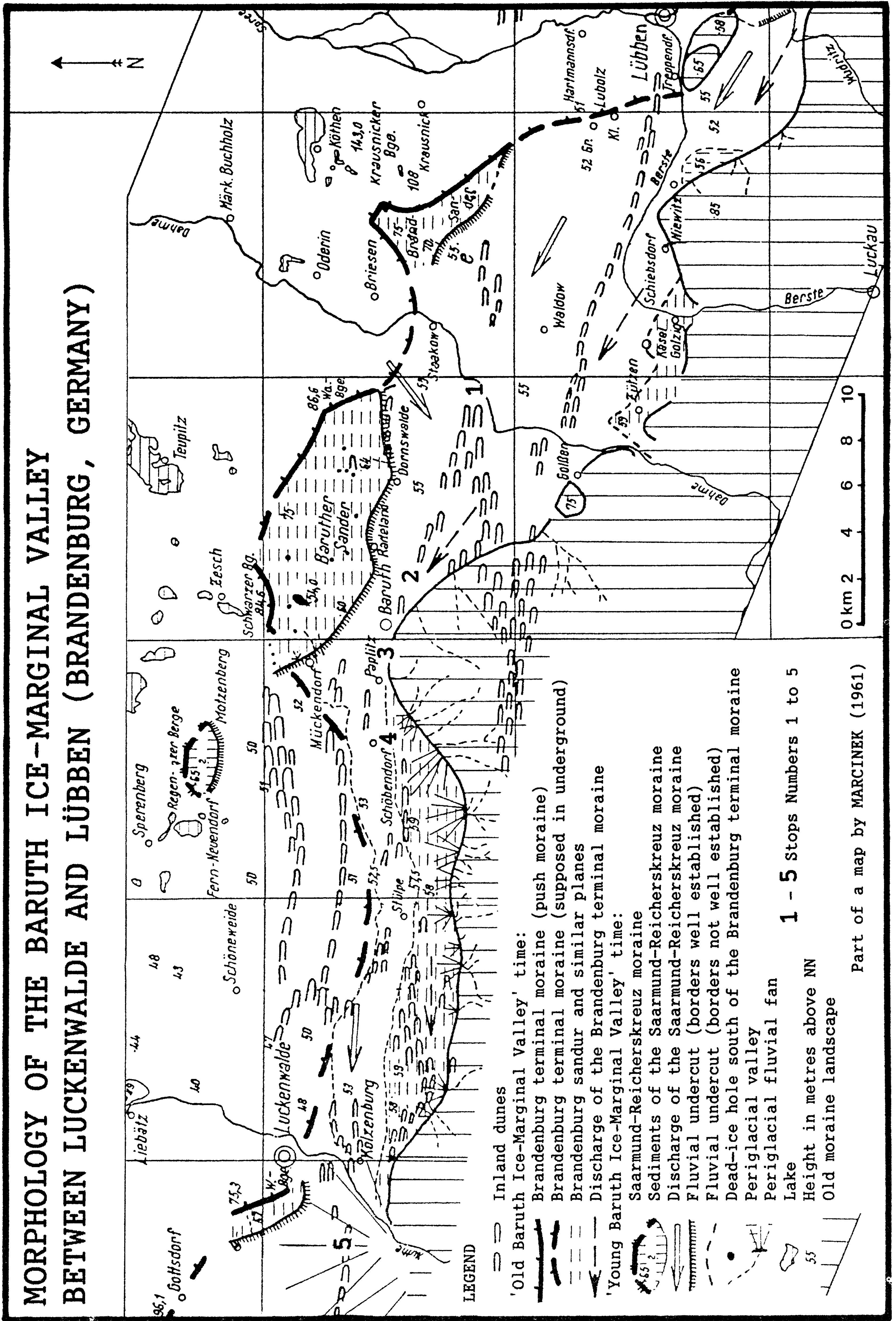
Abb. 1 Morphologie des Baruther Urstromtals zwischen Luckenwalde und Lübben (Brandenburg)
