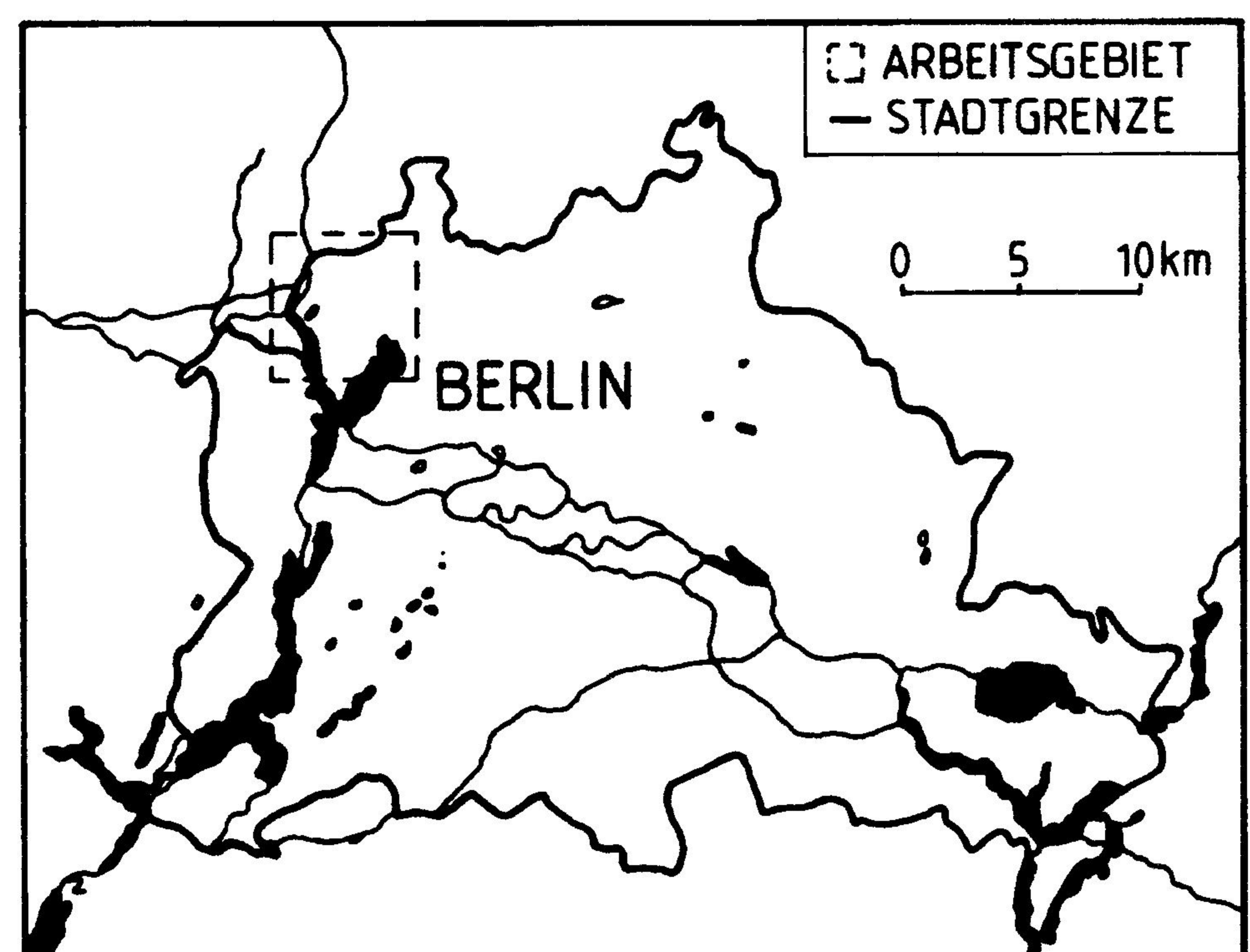
Abb. 1 Lage des Exkursionsgebietes (Abb. 2) im Berliner Stadtbereich (nach TESCHNER-STEINHARDT & MÜLLER 1994)
