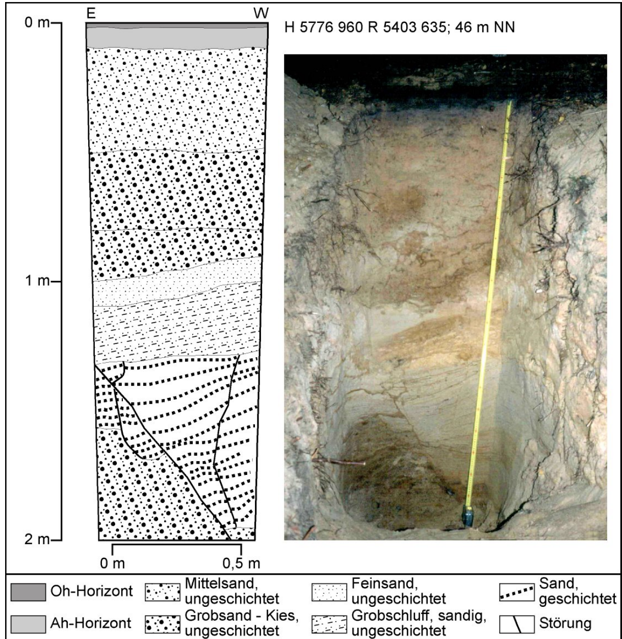
Abb. 84: Schurf ADQ6
