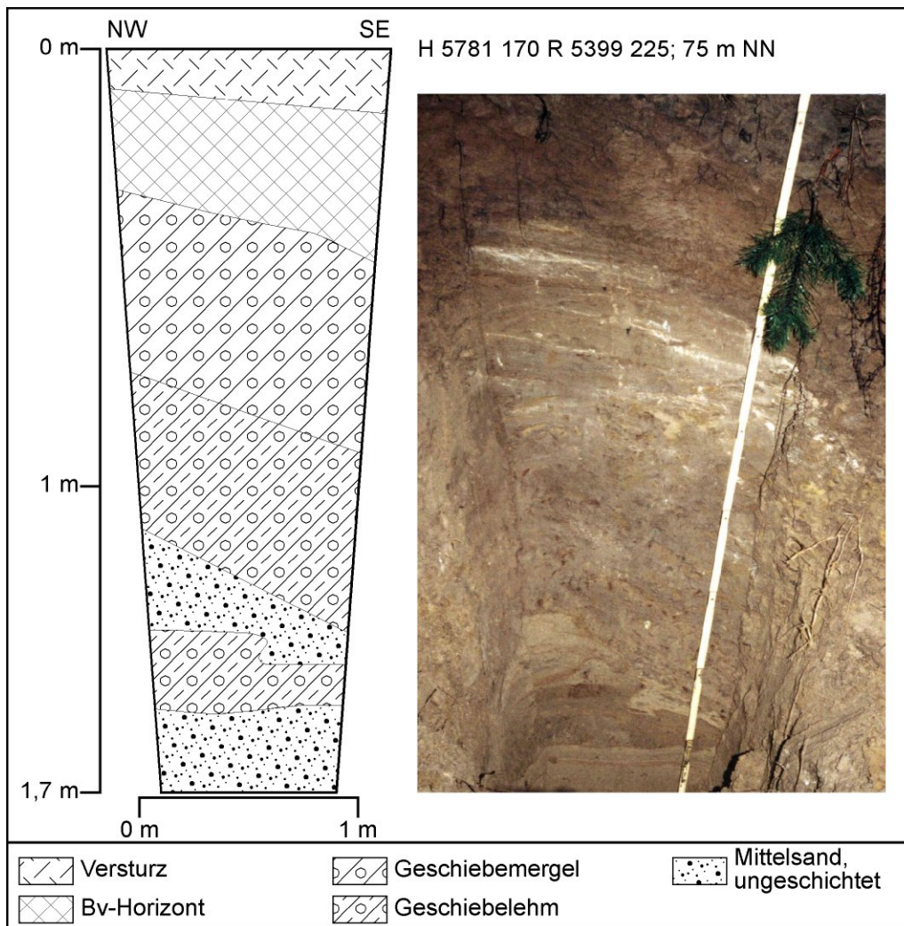
Abb. 125: Schurf Zehr1
