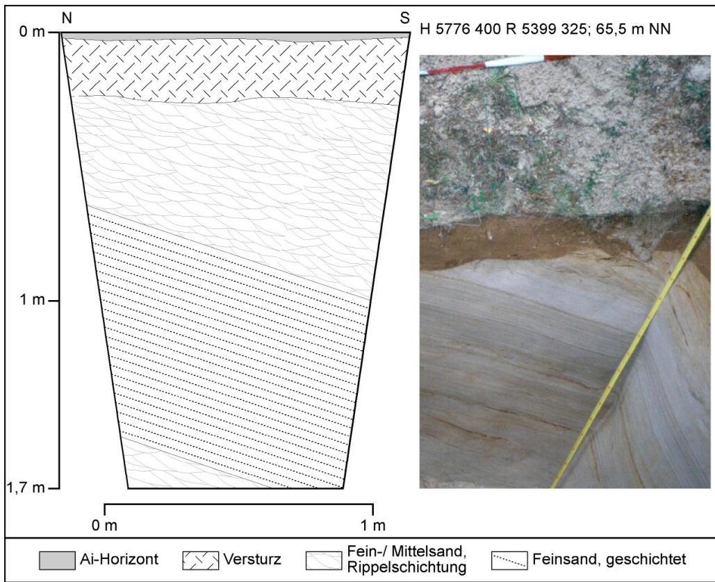
Abb. 131: Schurf Zesch6
