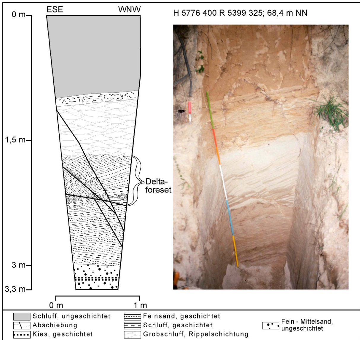
Abb. 128: Schurf Zesch1
