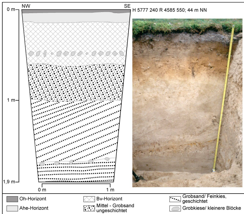
Abb. 120: Schurf SB1
