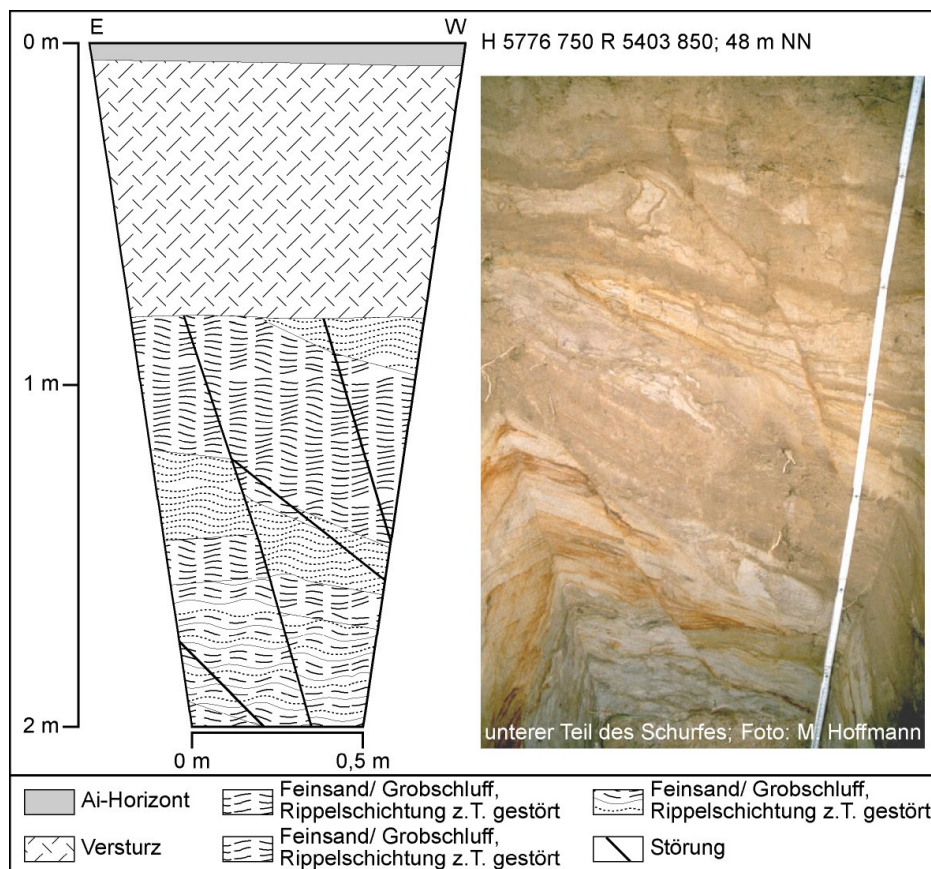
Abb. 87: Schurf Neu3
