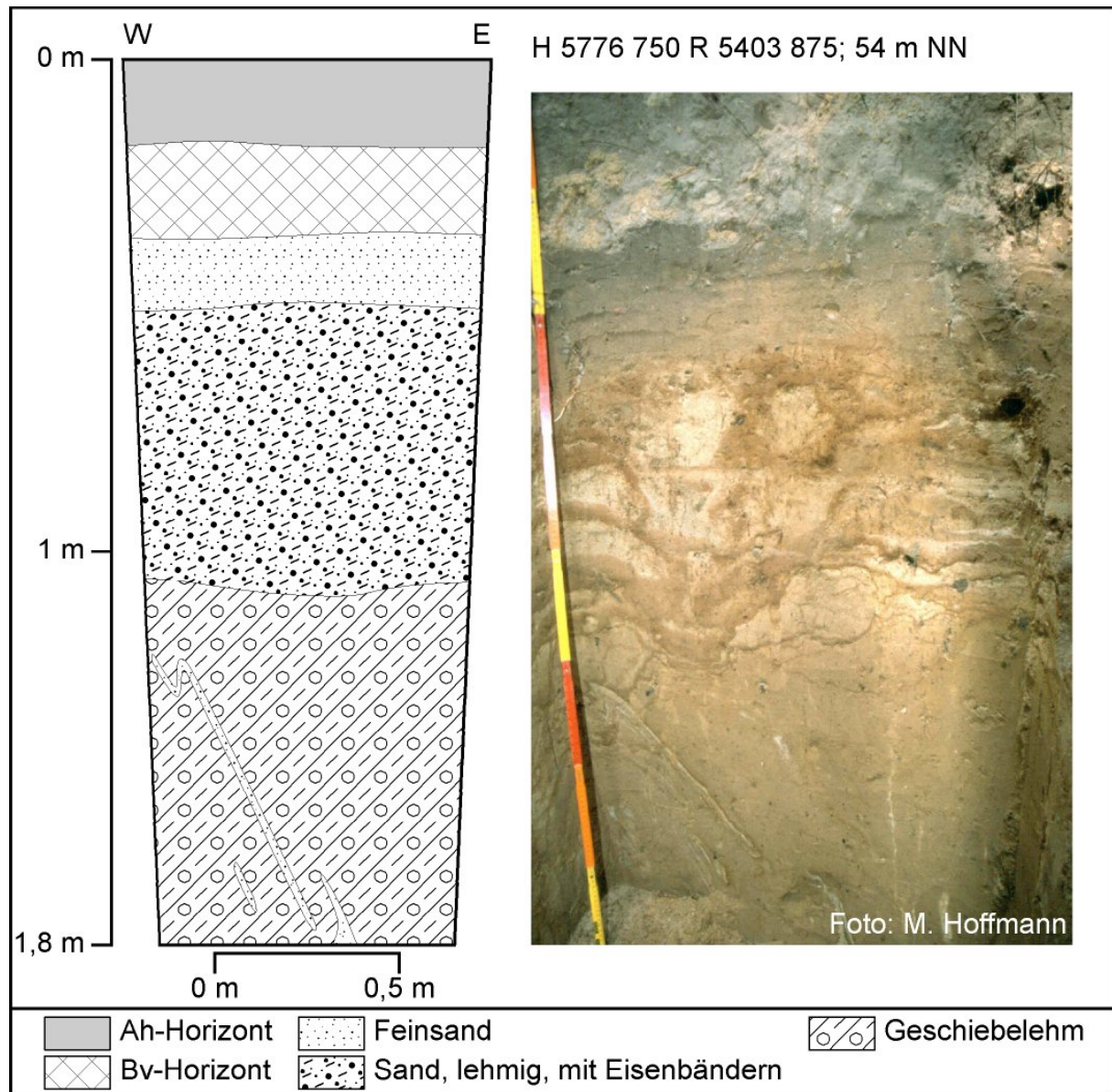
Abb. 85: Schurf Neu1
