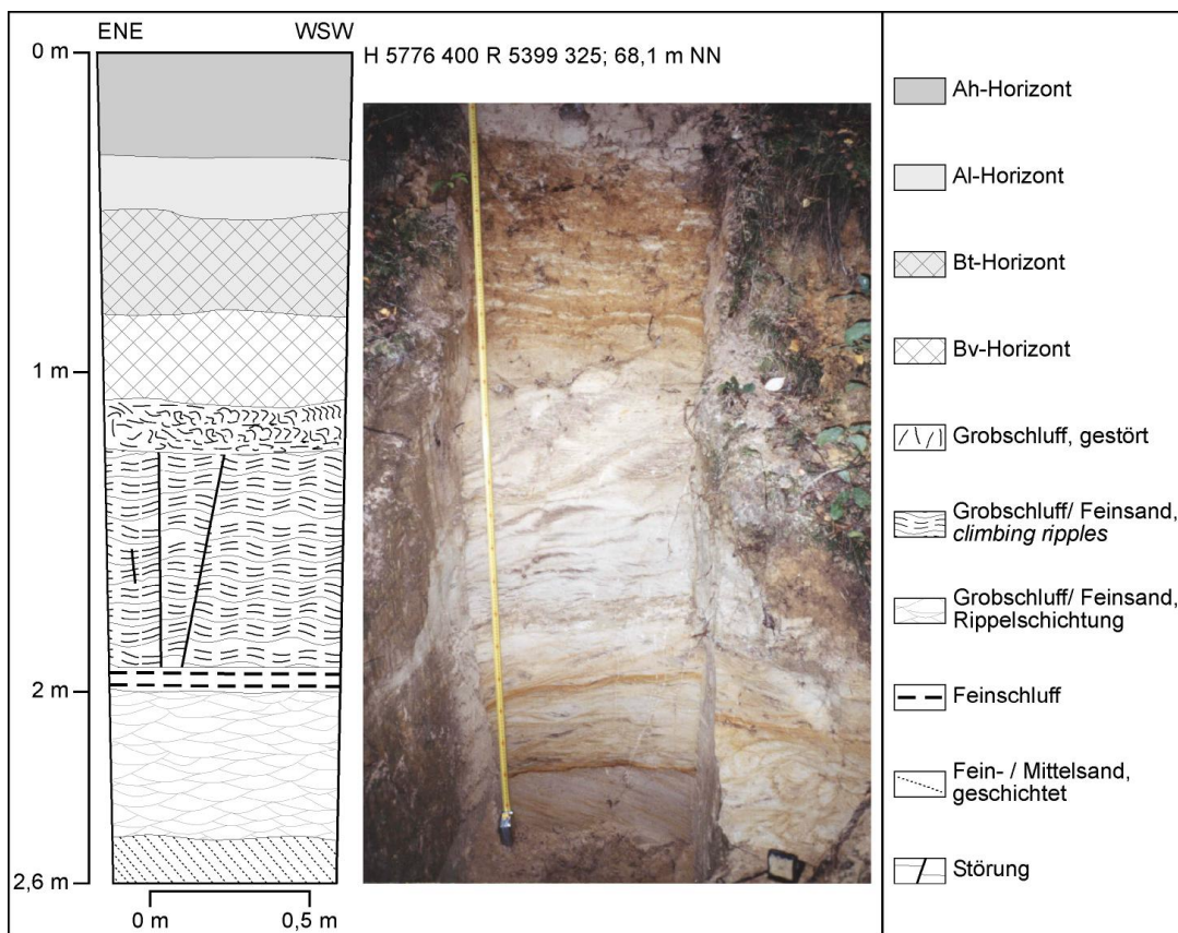
Abb. 132: Schurf Zesch7
