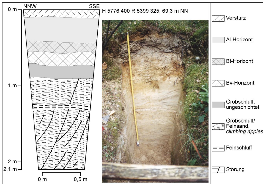
Abb. 134: Schurf Zesch9
